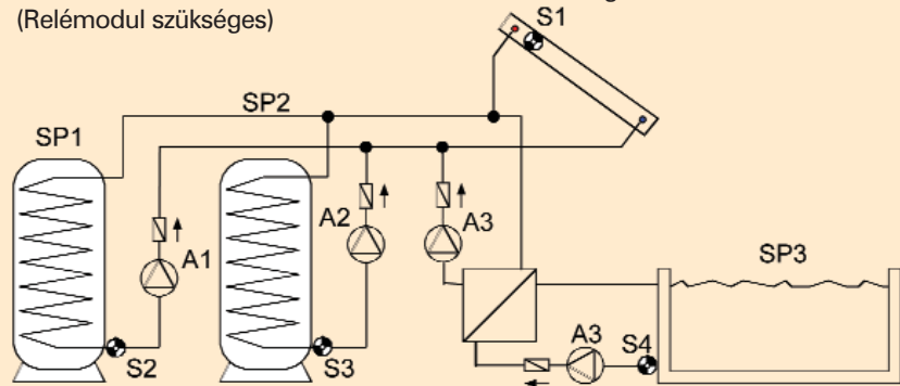
Szolárrendszer 2 tárolóval és medencefűtéssel - "Prog. 224" (Relémodul szükséges)
