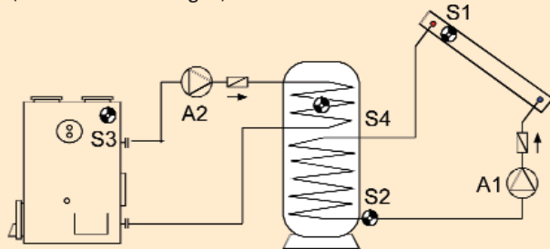
Egyszerű szolárrendszer termosztát funkcióval - "Prog. 80" (Relémodul szükséges)
