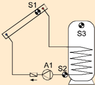
Egyszerű szolárrendszer - "Prog 0"
