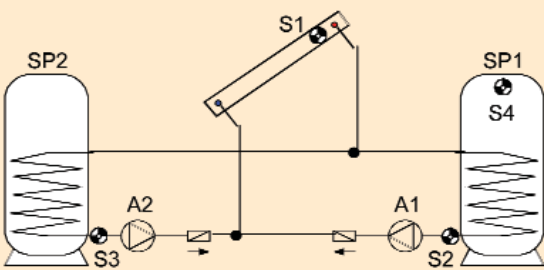
Szolárrendszer 2 tárolóval - "Prog. 48" (Relémodul szükséges)
