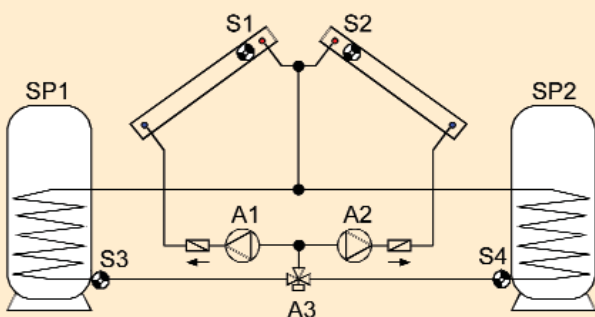
Szolárrendszer 2 kollektor felülettel, 2 tárolóval - "Prog. 240" (Relémodul szükséges)
