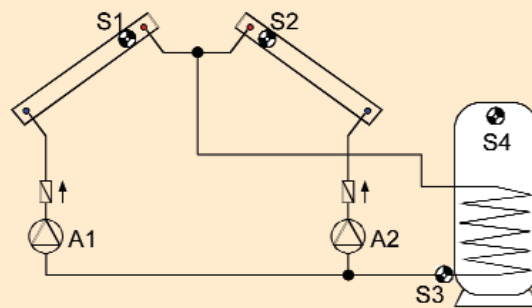
Szolárrendszer 2 kollektorfelülettel, egy tárolóval - "Prog. 64" (Relémodul szükséges)
